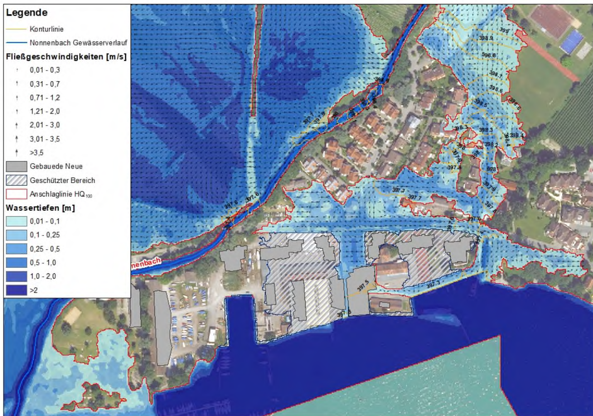
Abbildung 5-7 Wassertiefen und Fließgeschwindigkeiten im Untersuchungsbereich bei HQ 100 Nonnenbach und HQ 20 Bodensee im Planzustand mit naB und Hotel einschl. Berücksichtigung der Durchgängigkeit
