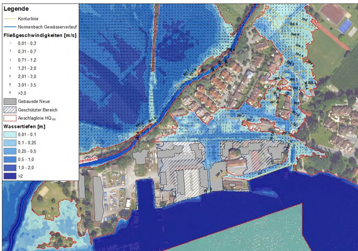
Abbildung 5-9 Wassertiefen und Fließgeschwindigkeiten im Untersuchungsbereich bei HQ 100 Nonnenbach und HQ 20 Bodensee im Planzustand mit naB und Hotel einschl. Berücksichtigung der Durchgängigkeit und Überarbeitung Bereich Seepark Kressbronn
