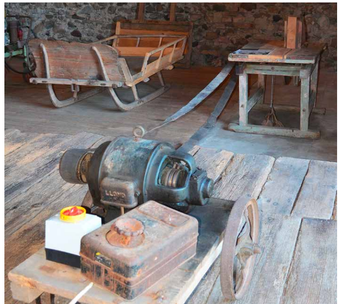
Frühes Strom-„Netz“: Der 1920 angeschaffte Elektromotor konnte über Flachriemen unter anderem auch die Kreissäge antreiben.
