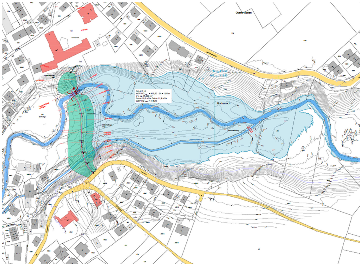
Planungsentwurf eines Rückhaltebeckens im Bochenloch
